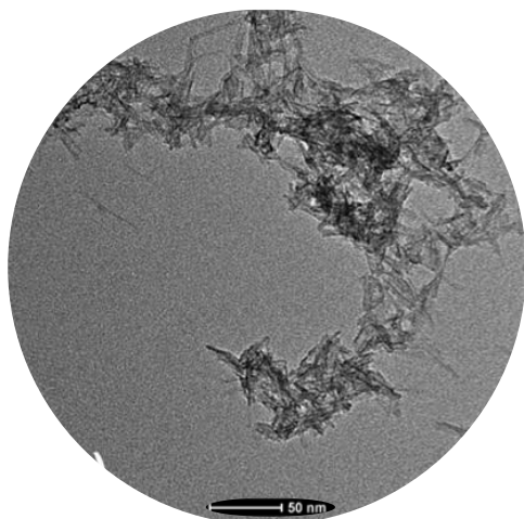
Imagem de Microscopia Eletrônica de Transmissão de nanofios de WO_x (a) baixa magnificação e (b) alta magnificação.
